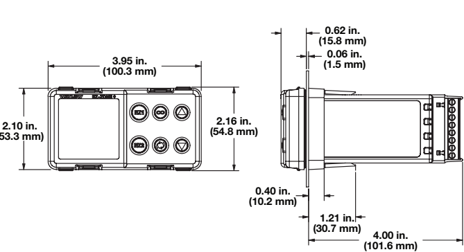
EZ-ZONE PM 1/8 DIN - Horizontal
