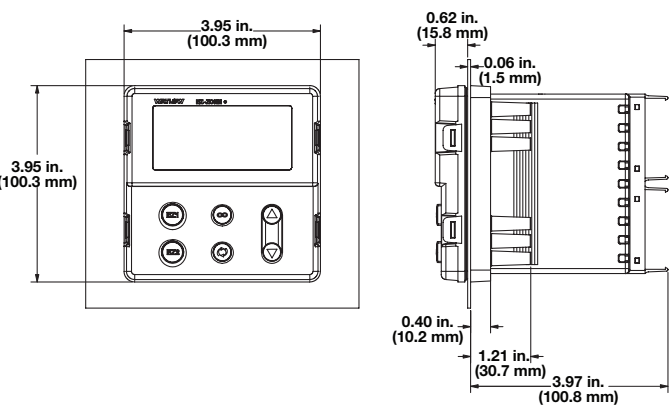
EZ-ZONE PM 1/4 DIN
